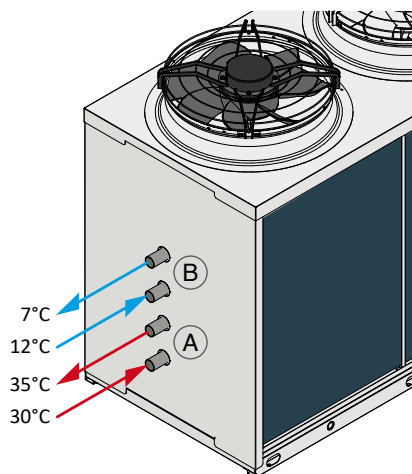
Raffreddamento + Riscaldamento acqua utenze
